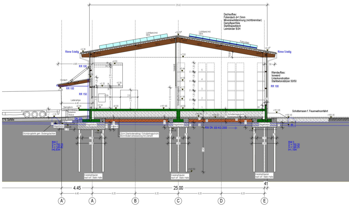
Schnitt A-A
