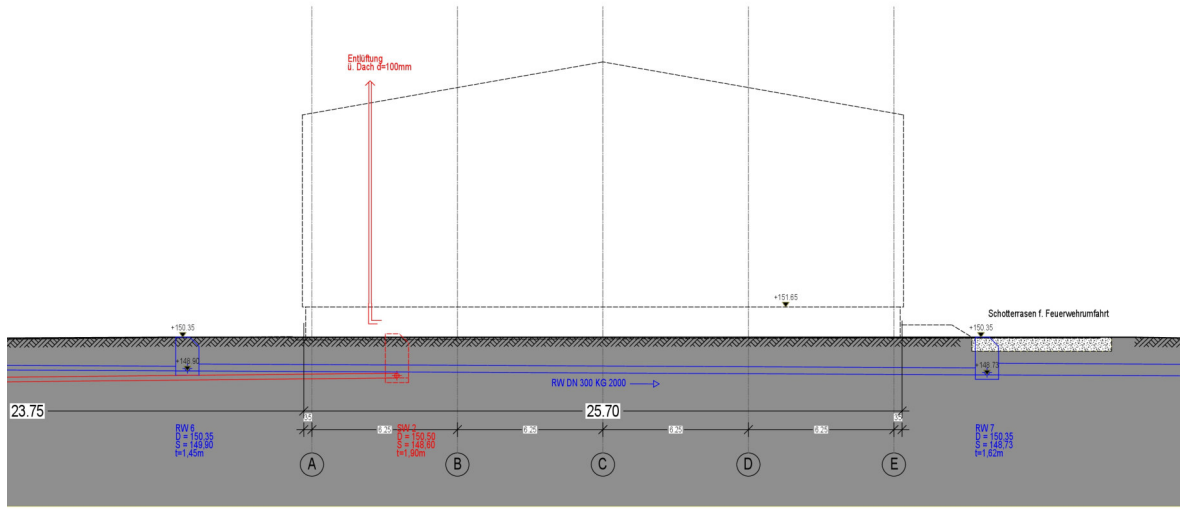
Schnitt B-B
